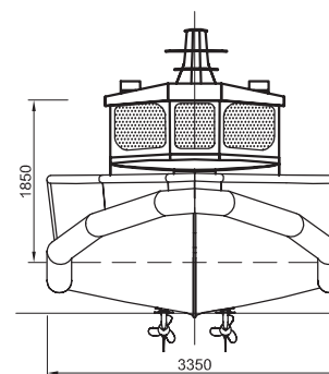
VISTA TRANSVERSAL (PROA)
