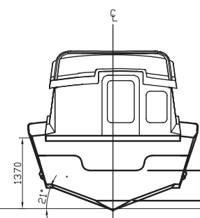
VISTA TRANSVERSAL (POPA)
