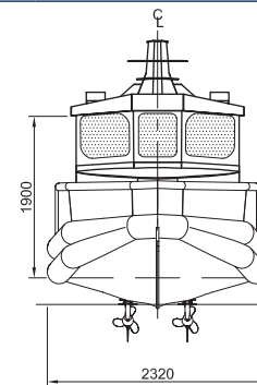
VISTA TRANSVERSAL (PROA)
