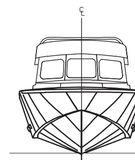
VISTA TRANSVERSAL (PROA)
