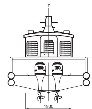
VISTA TRANSVERSAL (POPA)
