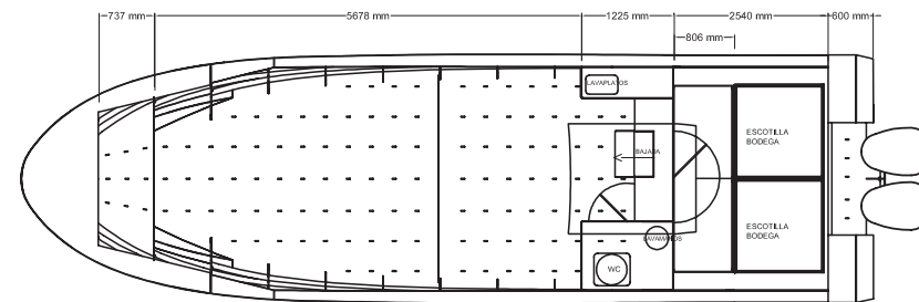
PLANO DE CUBIERTAS
