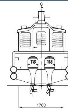
VISTA TRANSVERSAL (POPA)
